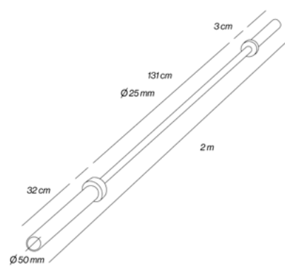
OLIMPIC BAR 2 M
